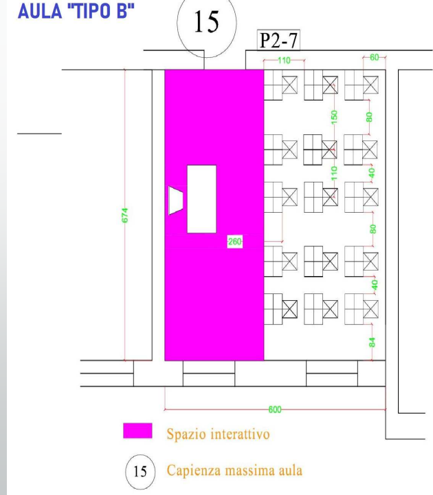
DISTRIBUZIONE ARREDI AULA "TIPO B"
